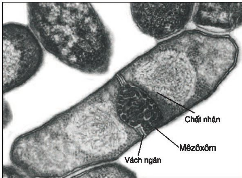
Hình 26.1. Hạt mêzôxôm của vi khuẩn dưới kính hiển vi điện tử
