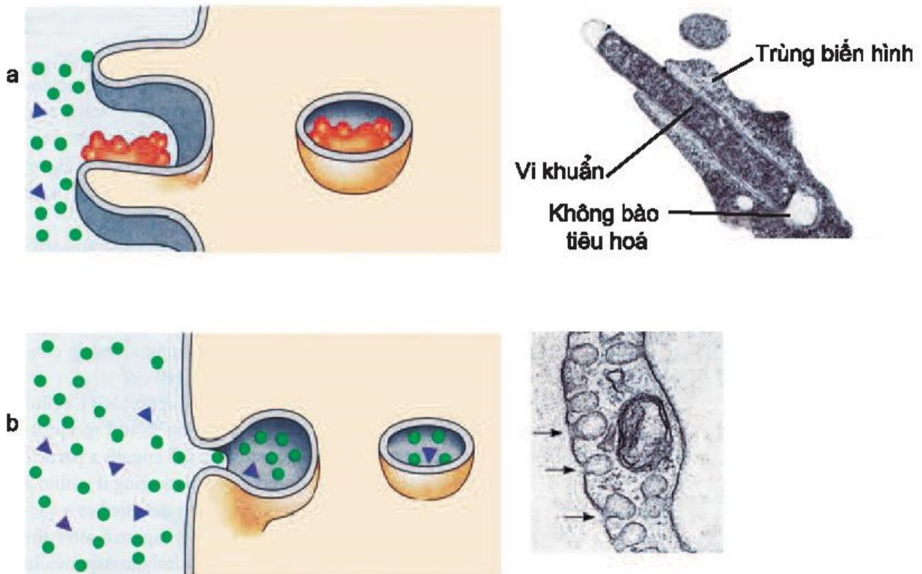
Hình 11.2. Sơ đồ quá trình thực bào và ẩm bào (bên trái là sơ đồ, bên phải là ảnh chụp dưới kính hiển vi điện tử)
