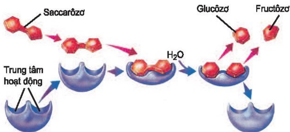
Hình 14.1. Sơ đồ mô tả cơ chế tác động của enzim saccharaza - một loại enzim phân huỷ đường saccarôzơ thành glucôzơ và fructôzơ
