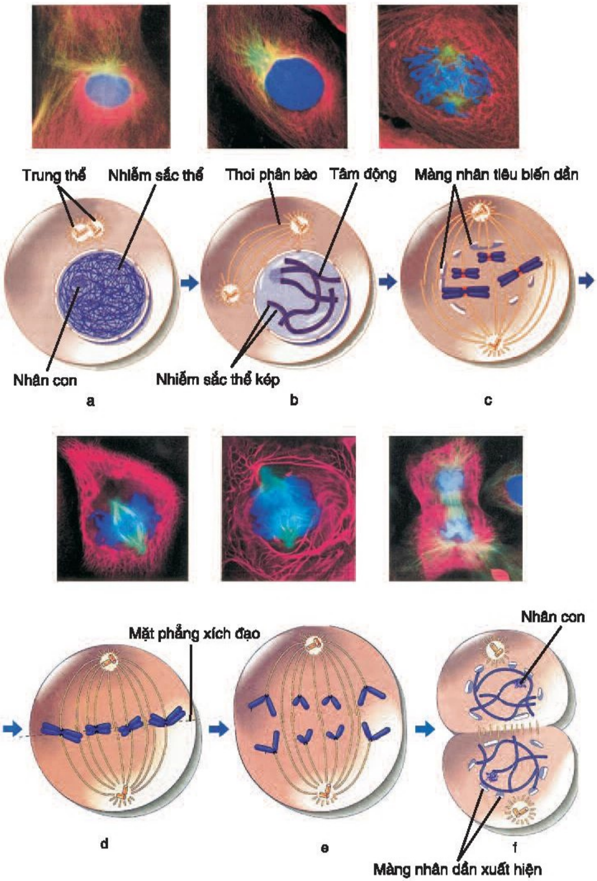
Hình 18.2. Nguyên phân ở tế bào động vật
