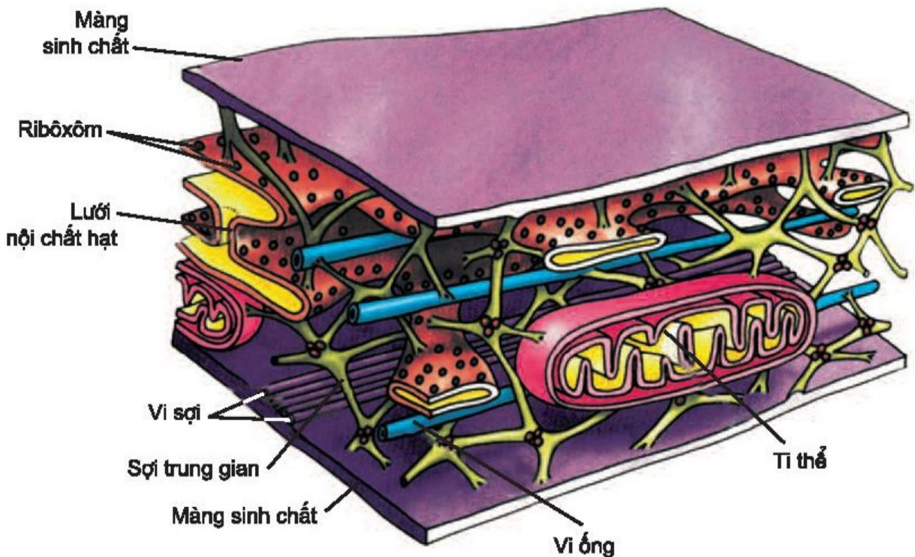
Hình 10.1. Khung xương tế bào
