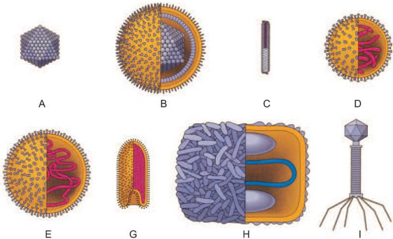
Hình 29.2. Hình thái của một số virus
