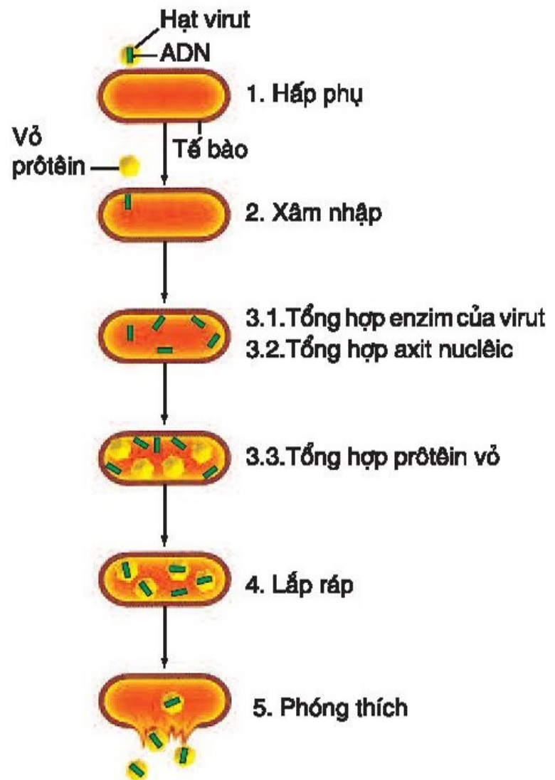
Hình 30. Chu trình nhân lên của phagơ
