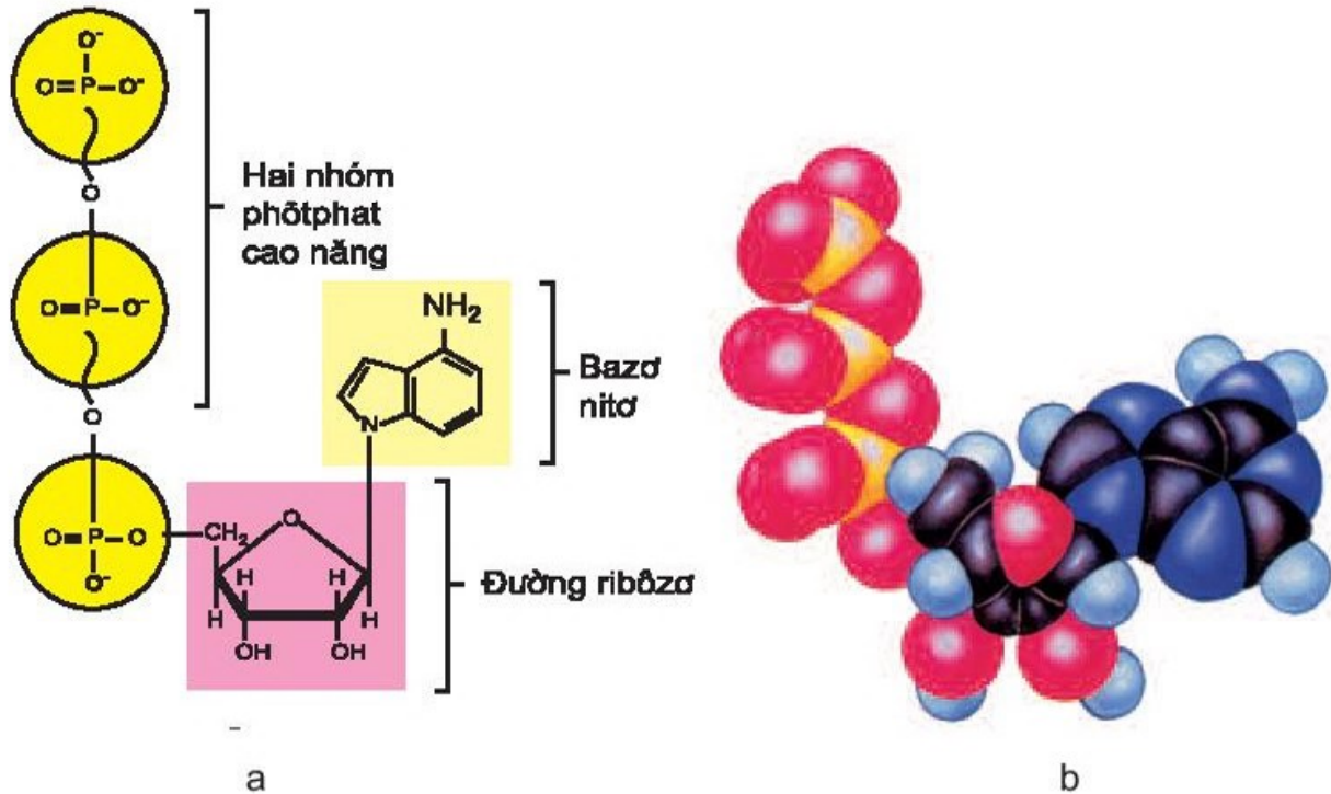
Hình 13.1. Cấu trúc của phân tử ATP
