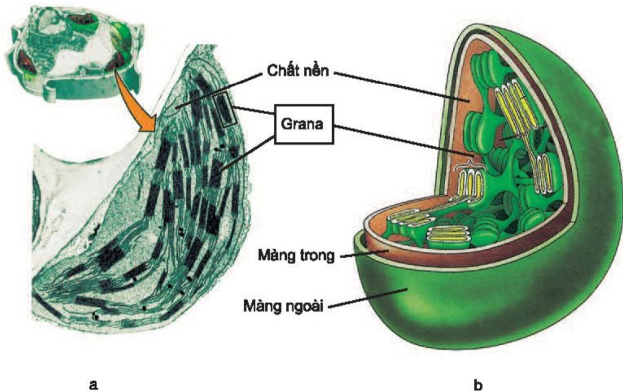
Hình 9.2. Cấu trúc của lục lạp
