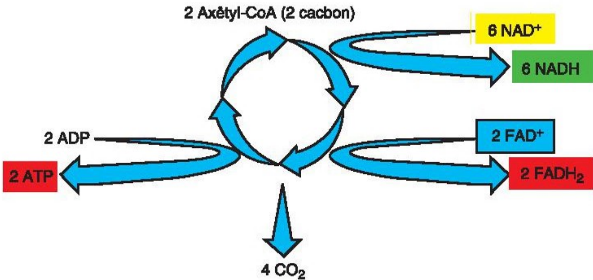
Hình 16.3. Sơ đồ tóm tắt chu trình Crep
