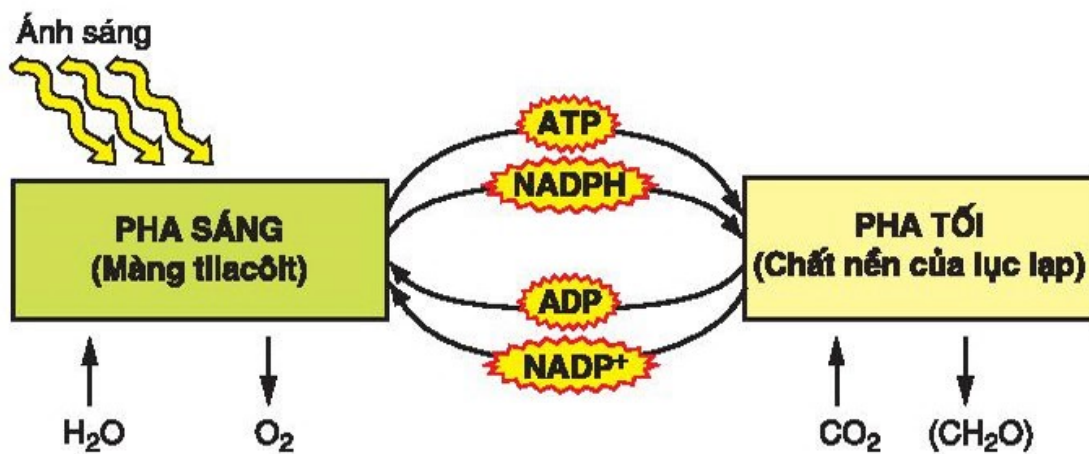
Hình 17.1. Hai pha của quá trình quang hợp
