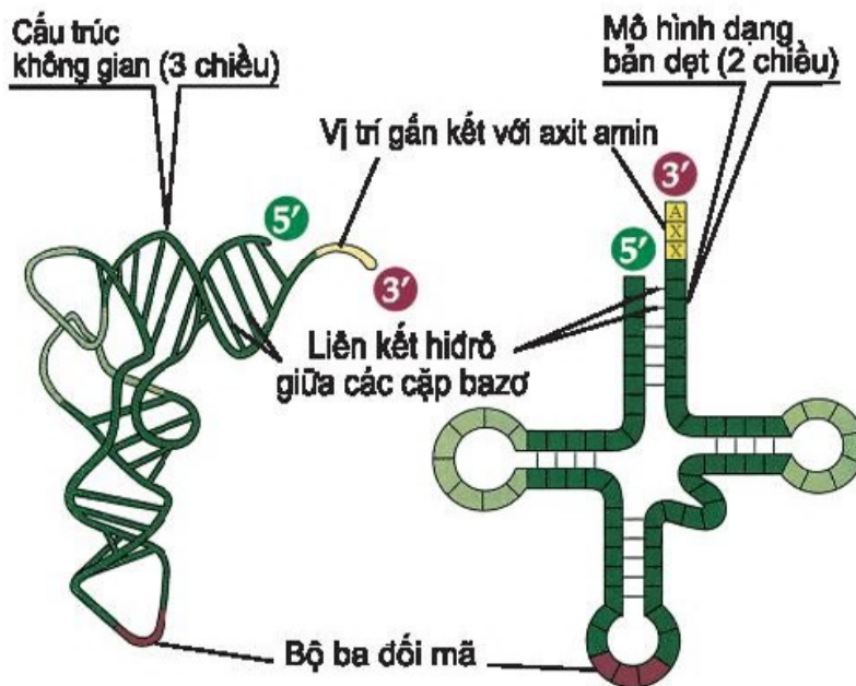
Hình 6.2. Mô hình cấu trúc của phân tử tARN
