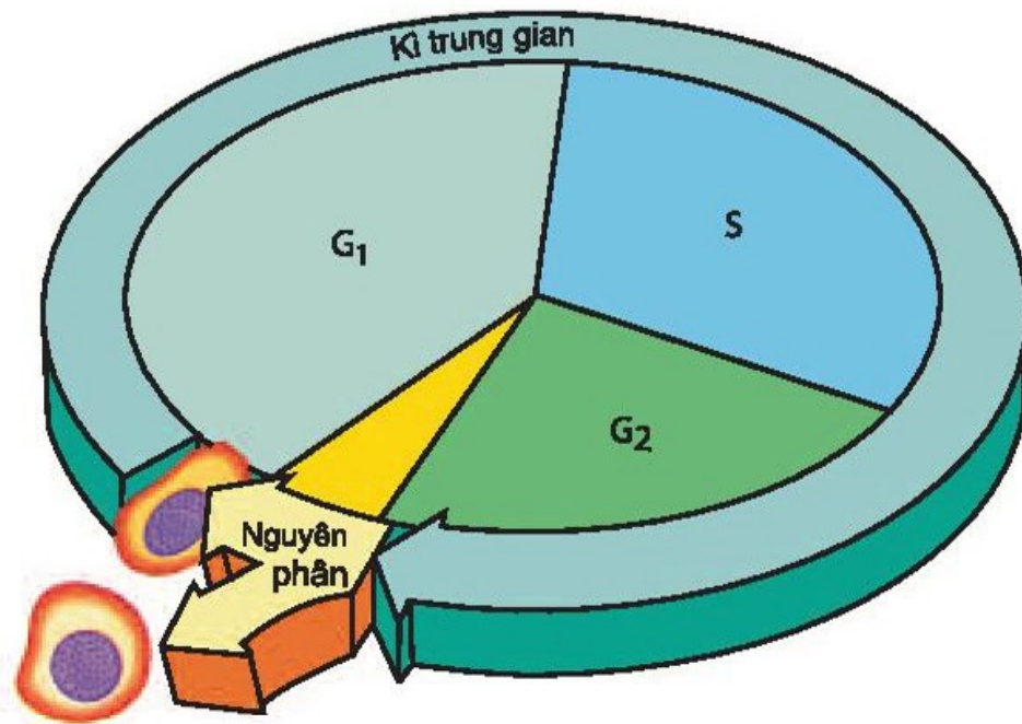
Hình 18.1. Chu kì tế bào
