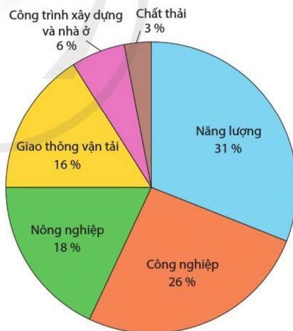
Hình 1.1. Biểu đồ tỉ lệ phát thải khí nhà kính trên thế giới theo lĩnh vực
