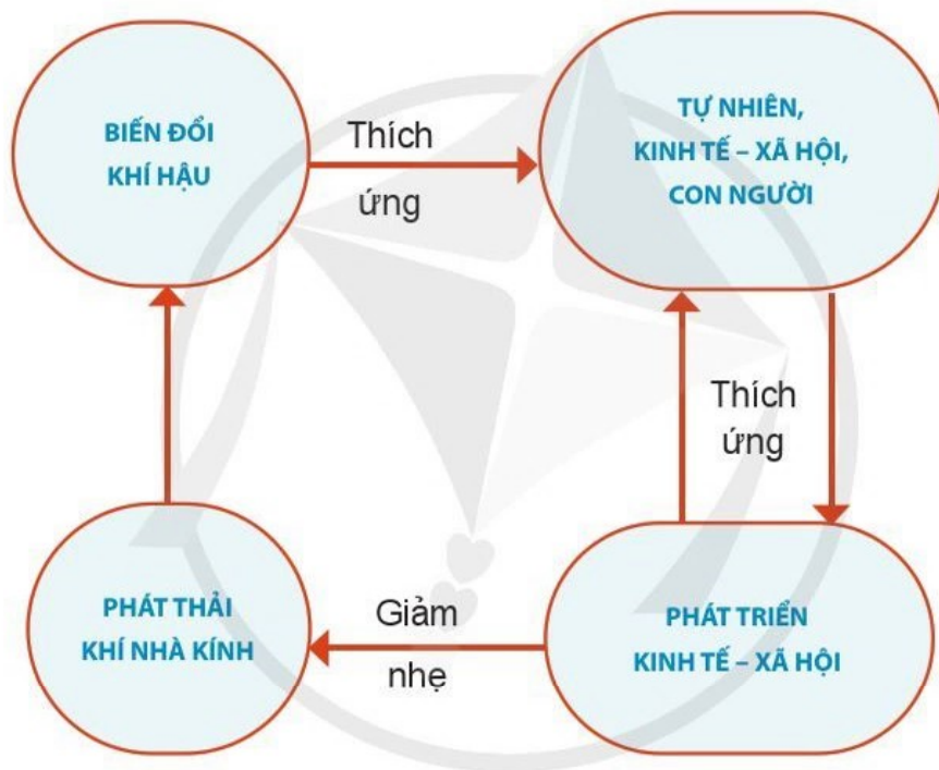
Hình 1.9. Sơ đồ ứng phó với biến đổi khí hậu
